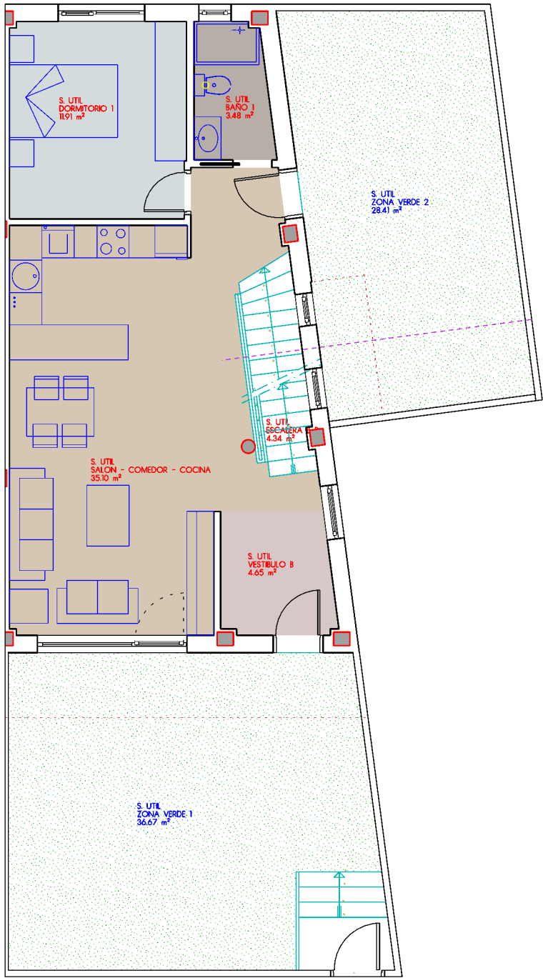
PLANTA BAJA
